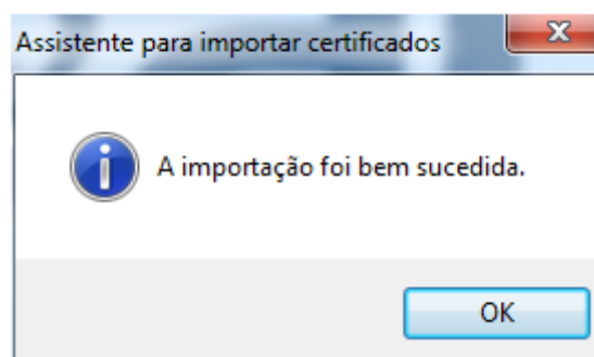
Figura 14 - Importação bem-sucedida.
