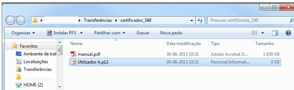
Figura 7 - Certificado extraído.
