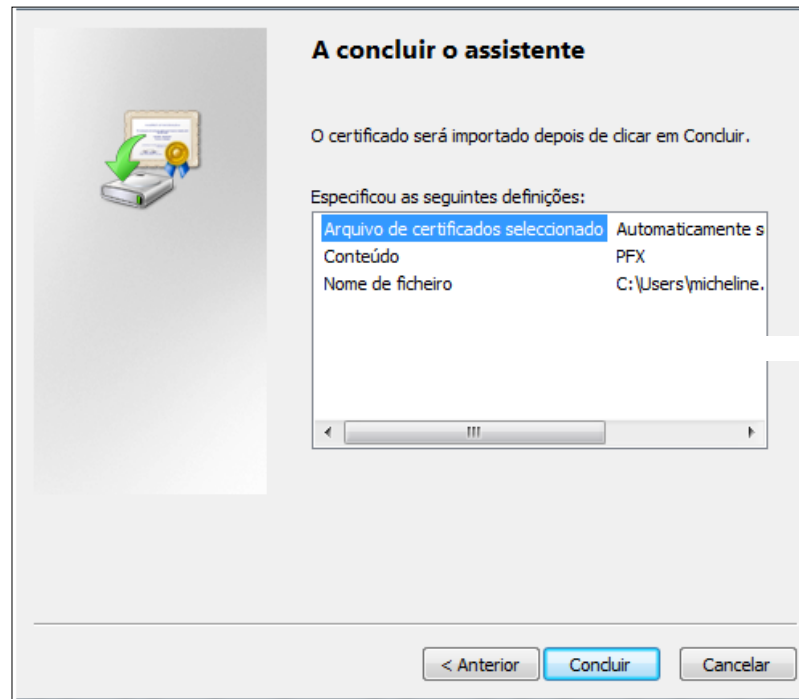
Figura 13 - Concluir instalação.
