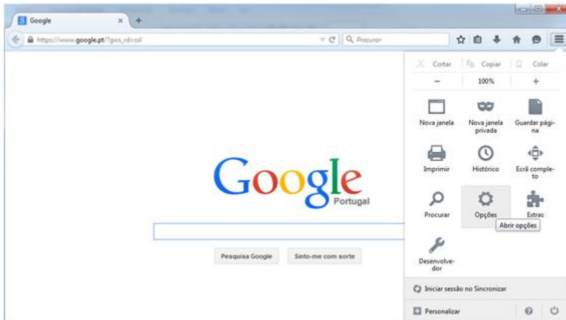
Figura 15 - Mozilla Firefox.
