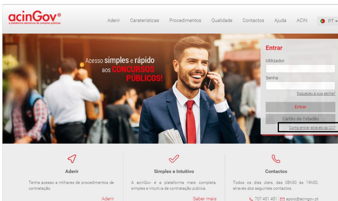
Figura 27 - acinGov.
