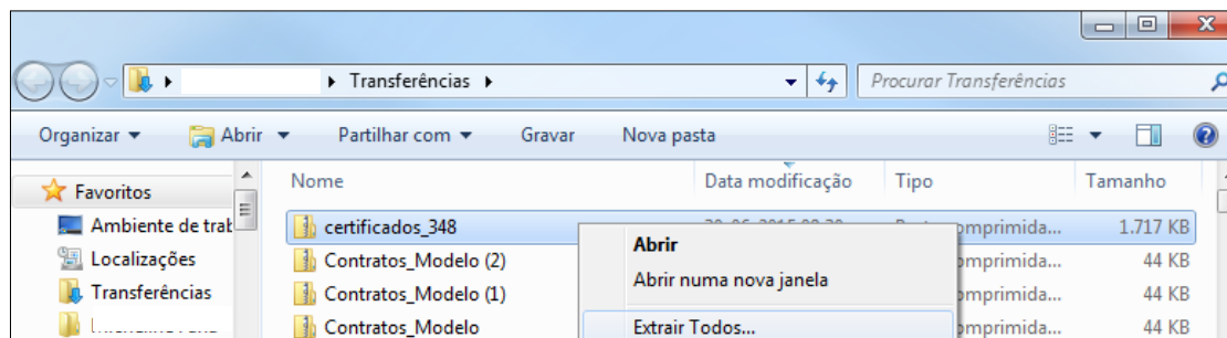
Figura 5 - Extrair ficheiro.
