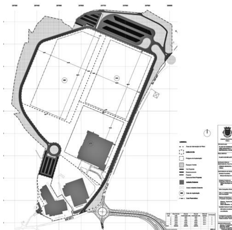
Figura 1 Plano de Pormenor da Área Industrial e Empresarial de Sinde/Tábua. Planta Síntese.
